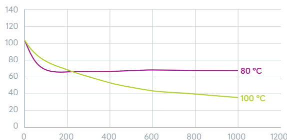
% de resistencia inicial = f (tiempo de exposición [horas])
